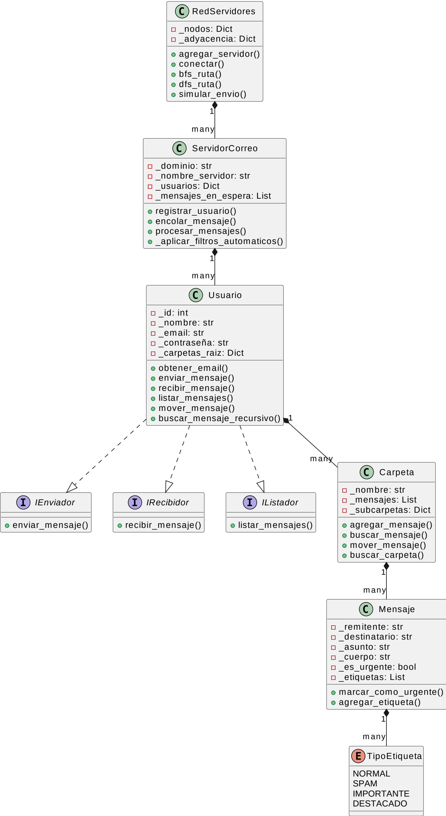
Diagrama de Clases del Sistema de Correo
